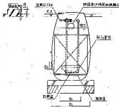
C—C'断面图
