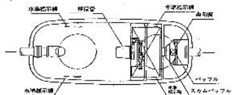
B—B'断面图
