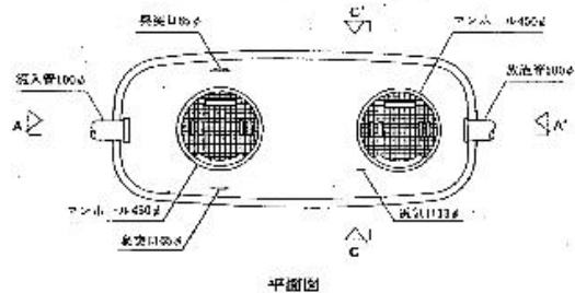
平衡图
