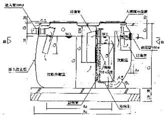
A—A 斷面圖
