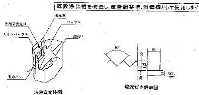
消毒室立体图
